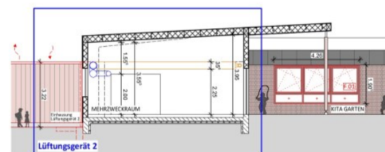
Schnitt C-C mit Ansicht West 1:100
