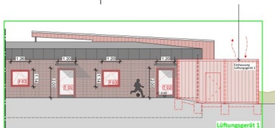
Ansicht Ost 1:100
